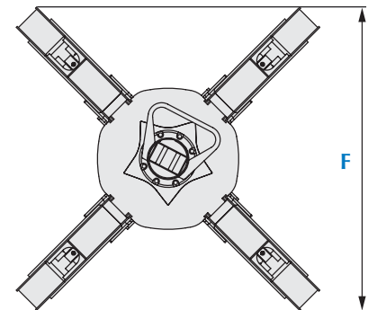
Encombrement version 4 griffes.
